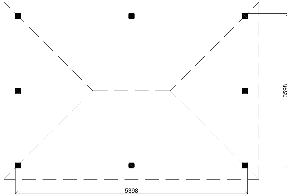
Plattegrond / Plan
