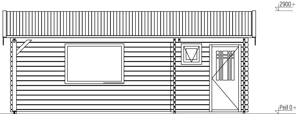
Vooraanzicht / Front view / Vorderansicht
